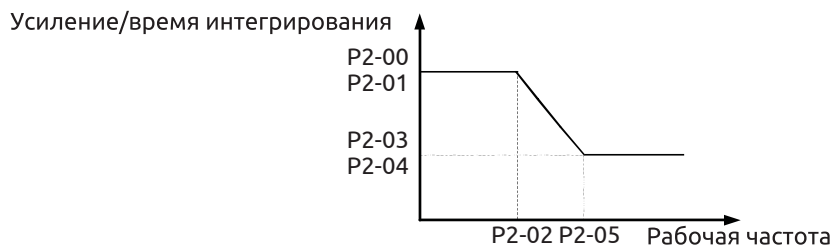
Диаграмма параметров контура скорости
