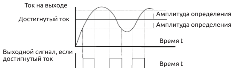
Схема функции достигнутого тока и достигнутой частоты
